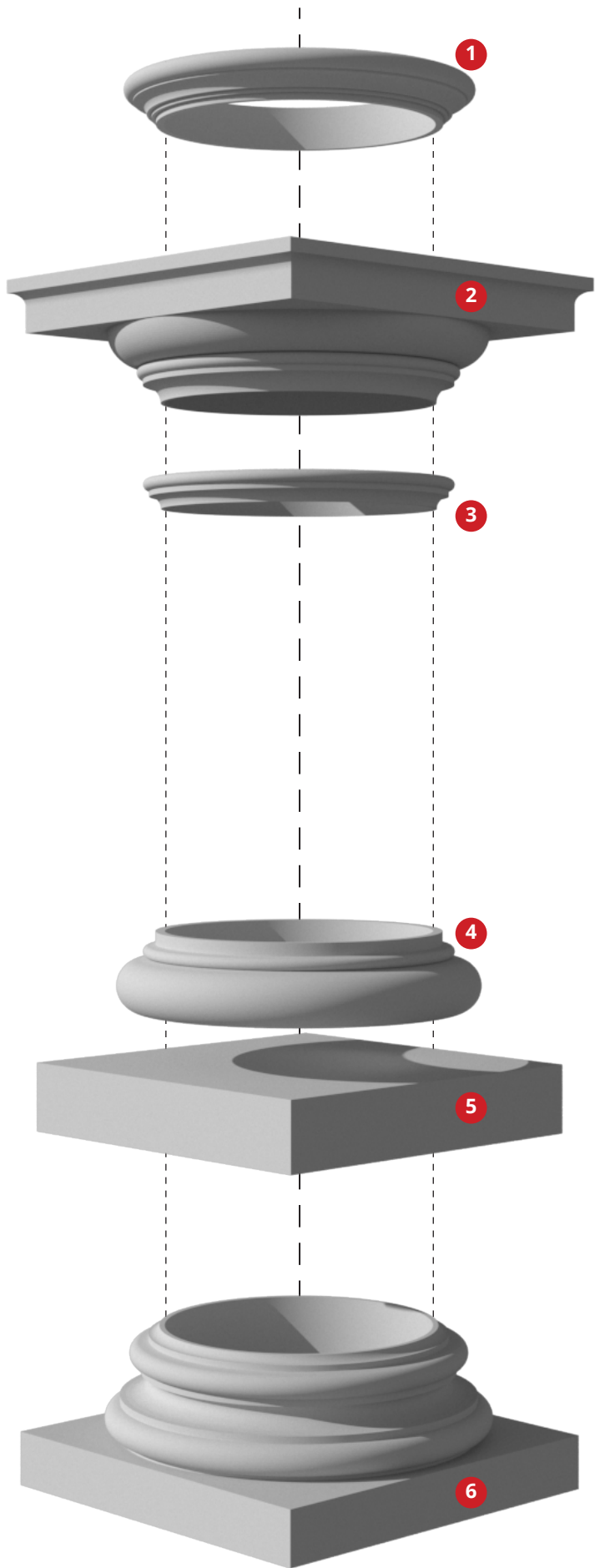
1. TUSCAN TORUS | TORT195 ( \varnothing 258x32mm)
